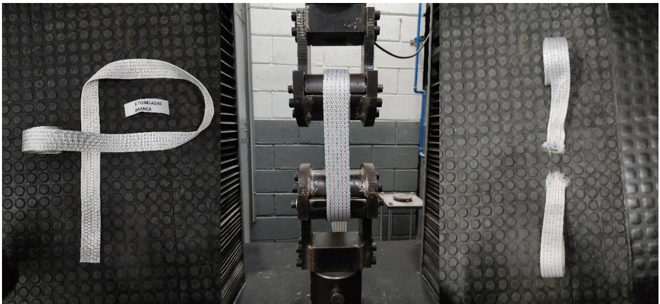
Foto nº 01 – Amostra antes do ensaio.
